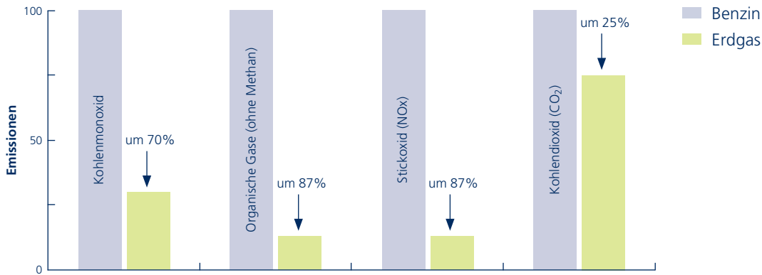
GRAFIK: REDUKTION DER ABGASEMISSIONEN DURCH ERDGAS
